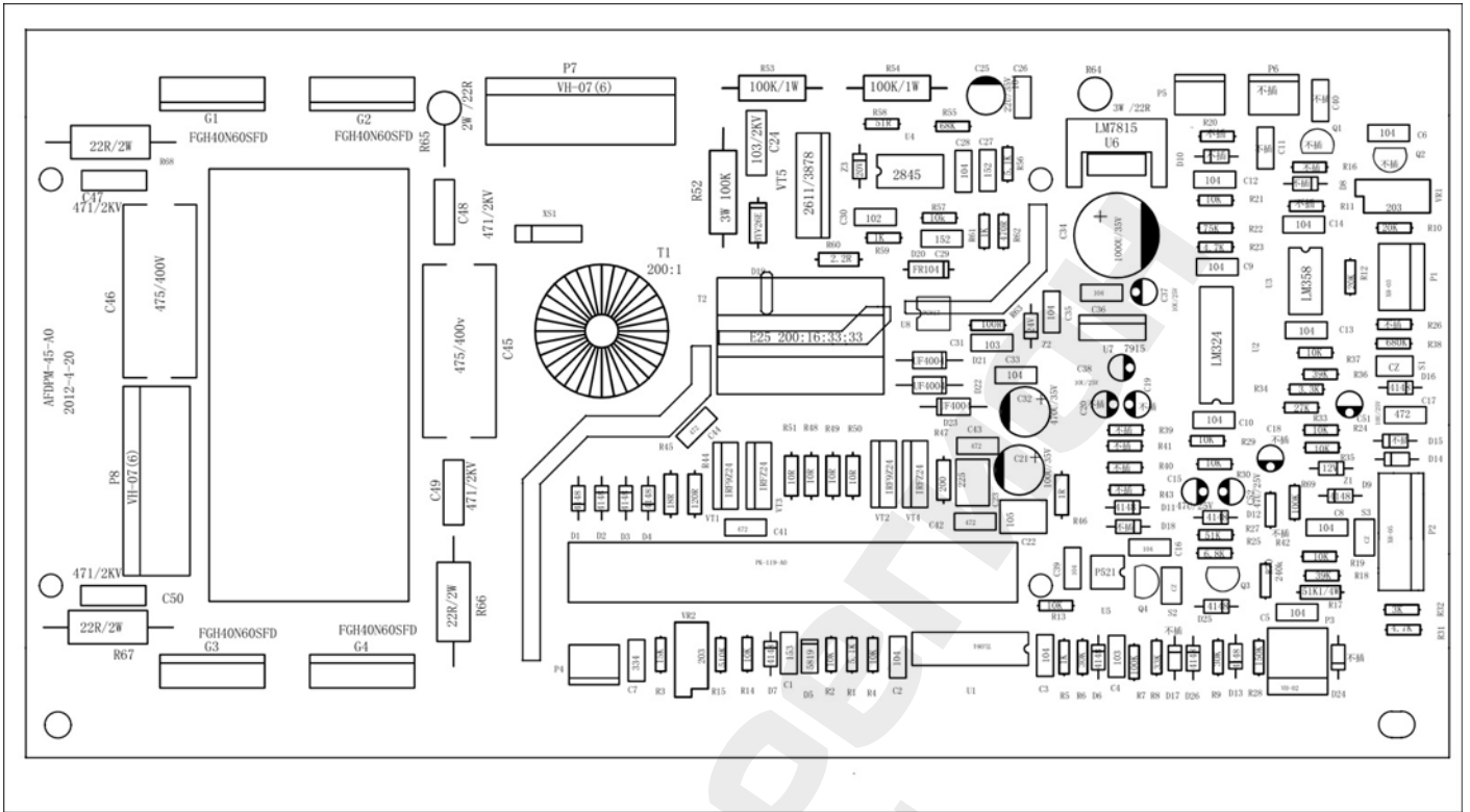
Плата средняя
