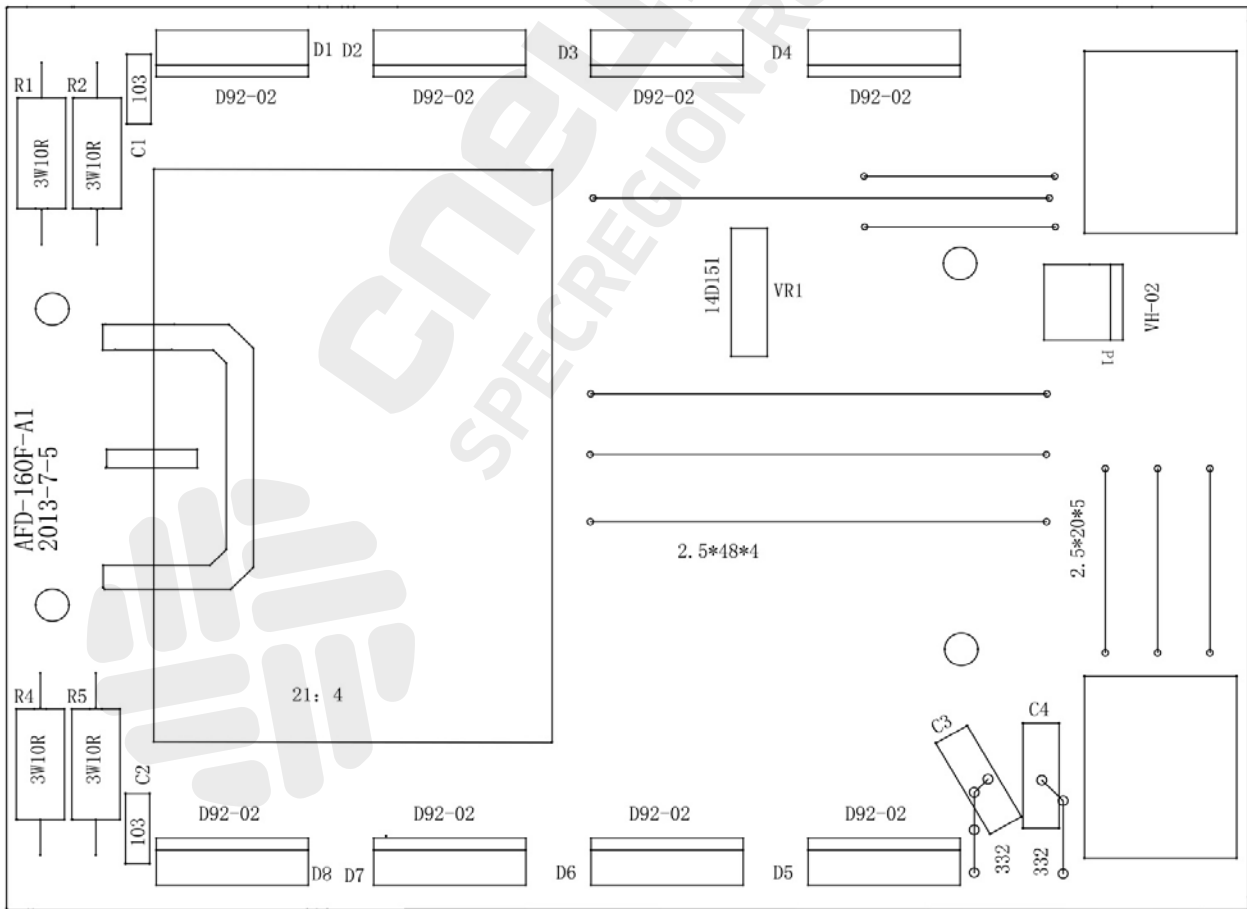
Плата средняя
